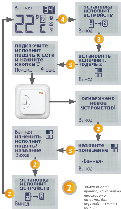
Рис. 28. Схема подключения дополнительных модулей к системе TP 820
